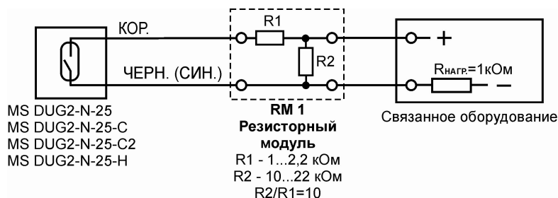
Схема подключения к связанному оборудованию
